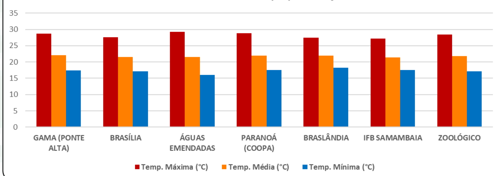
TEMPERATURAS MÉDIAS (DF) - MARÇO 2021
