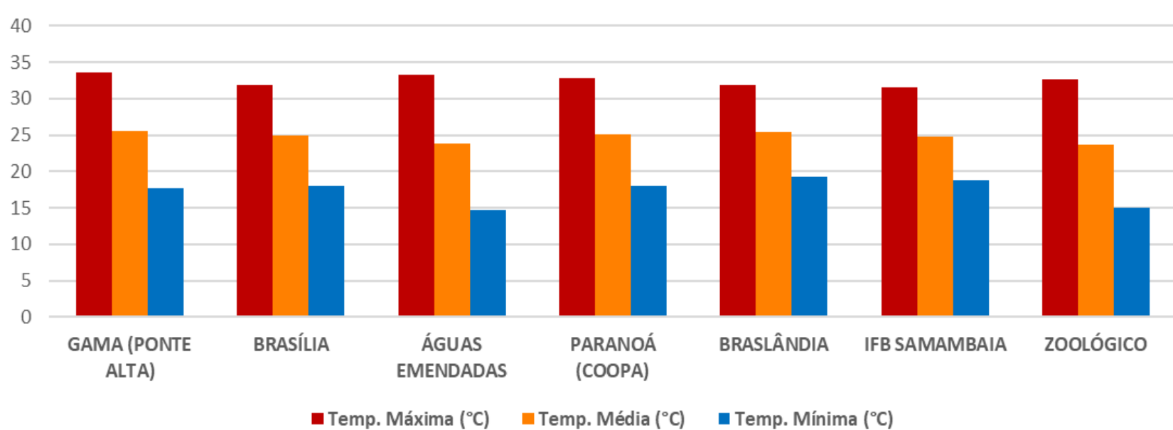
TEMPERATURAS MÉDIAS (DF) - SETEMBRO 2021
