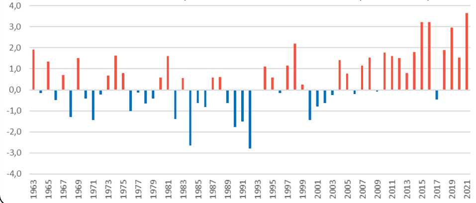
Anomalia de Temperatura Mínima - Setembro (1963-2021)
