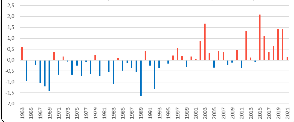
Anomalia de Temperatura Média - Dezembro (1963-2021)
