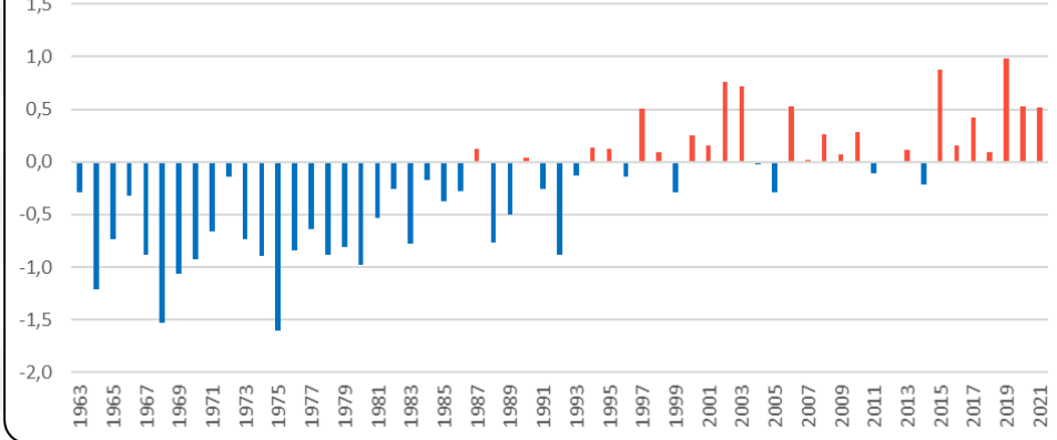
Anomalia de Temperatura Mínima - Dezembro (1963-2020)
