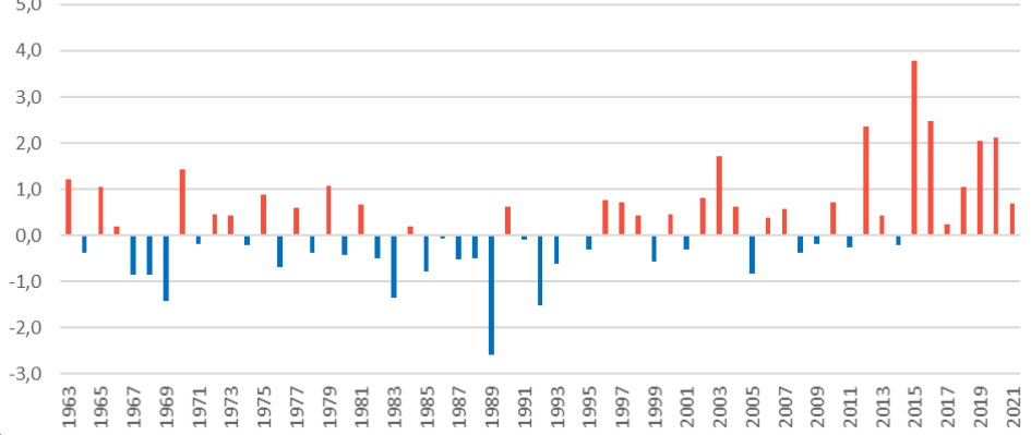
Anomalia de Temperatura Máxima - Dezembro (1963-2021)
