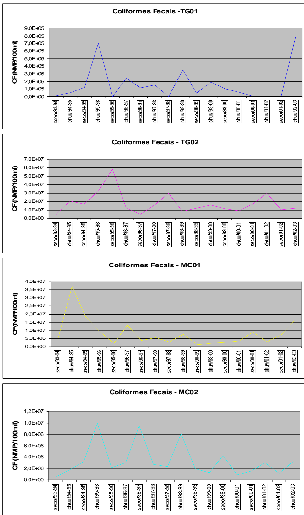
Figura 15 - Resultados de qualidade da água - CF, para os pontos monitorados - Períodos seco e chuvoso 1992 a 2003.
