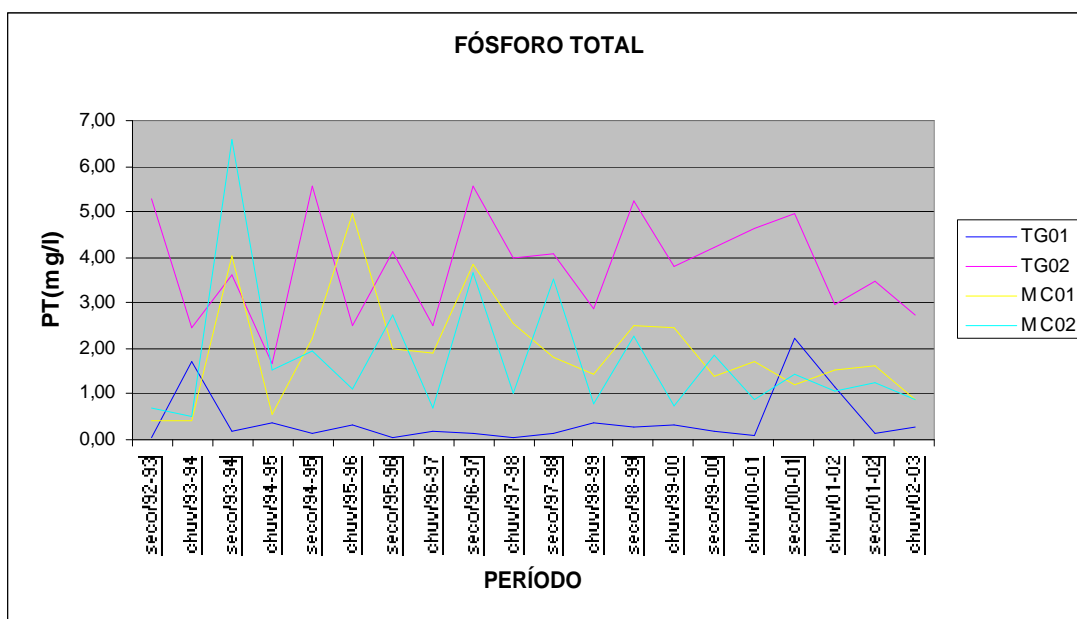
Figura 13 - Resultados de qualidade da água – PT, para os pontos monitorados - Períodos seco e chuvoso 1992 a 2003.
