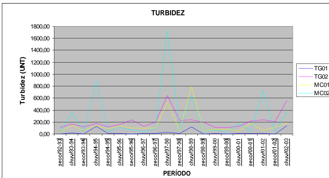
Figura 14 - Resultados de qualidade da água – Turbidez, para os pontos monitorados - Períodos seco e chuvoso 1992 a 2003.
