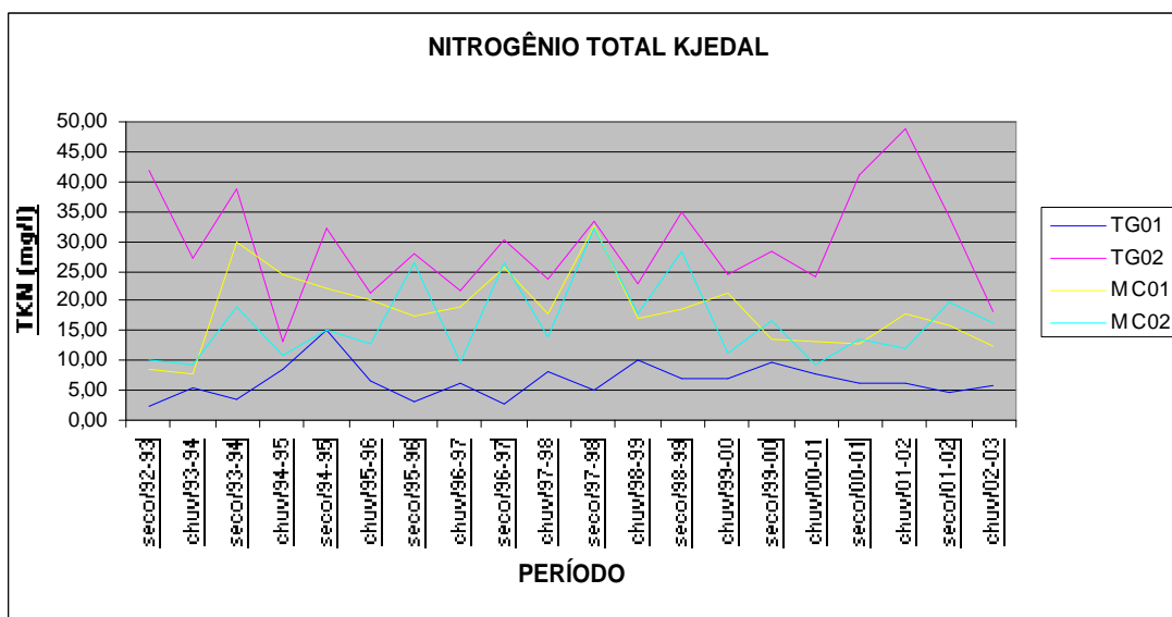
Figura 12 - Resultados de qualidade da água – TKN, para os pontos monitorados - Períodos seco e chuvoso 1992 a 2003.
