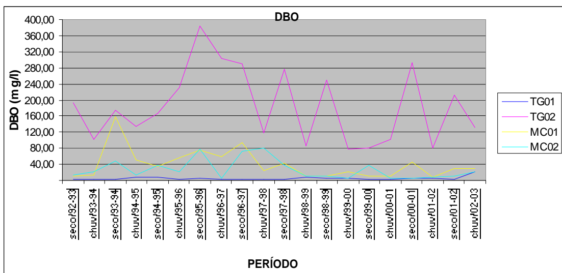
Figura 10 - Resultados de qualidade da água - DBO, para os pontos monitorados - Períodos seco e chuvoso 1992 a 2003. Fonte: Ribeiro, 2001
