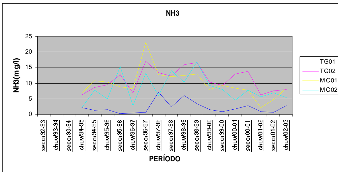
Figura 11 - Resultados de qualidade da água – NH 3 , para os pontos monitorados - Períodos seco e chuvoso 1992 a 2003.
