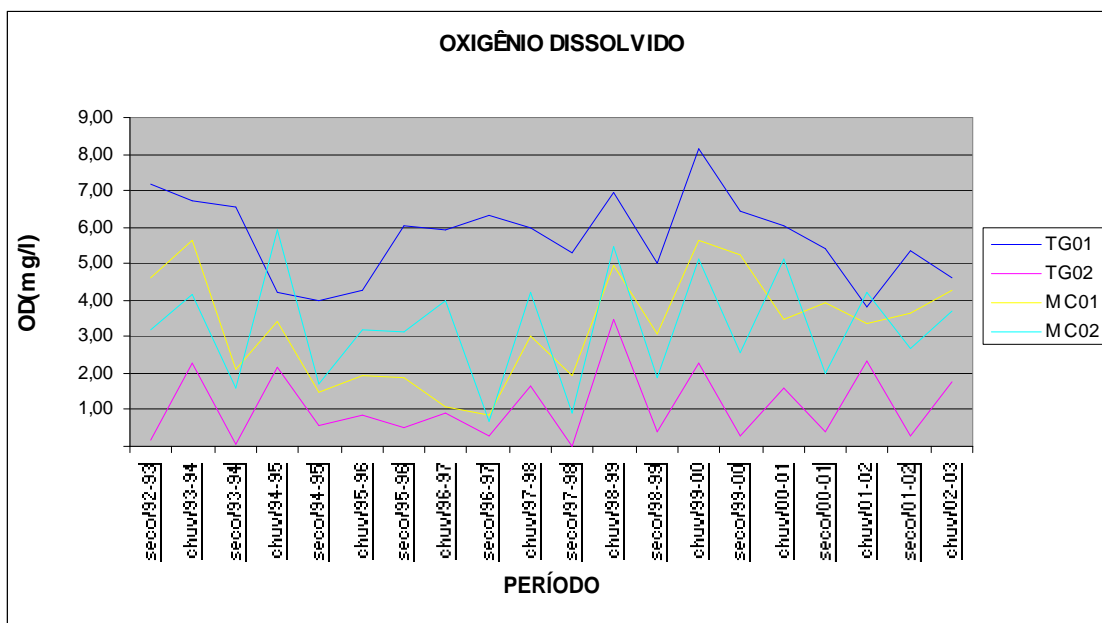
Figura 09 - Resultados de qualidade da água - OD, para os pontos monitorados - Períodos seco e chuvoso 1992 a 2003. Fonte: Ribeiro, 2001
