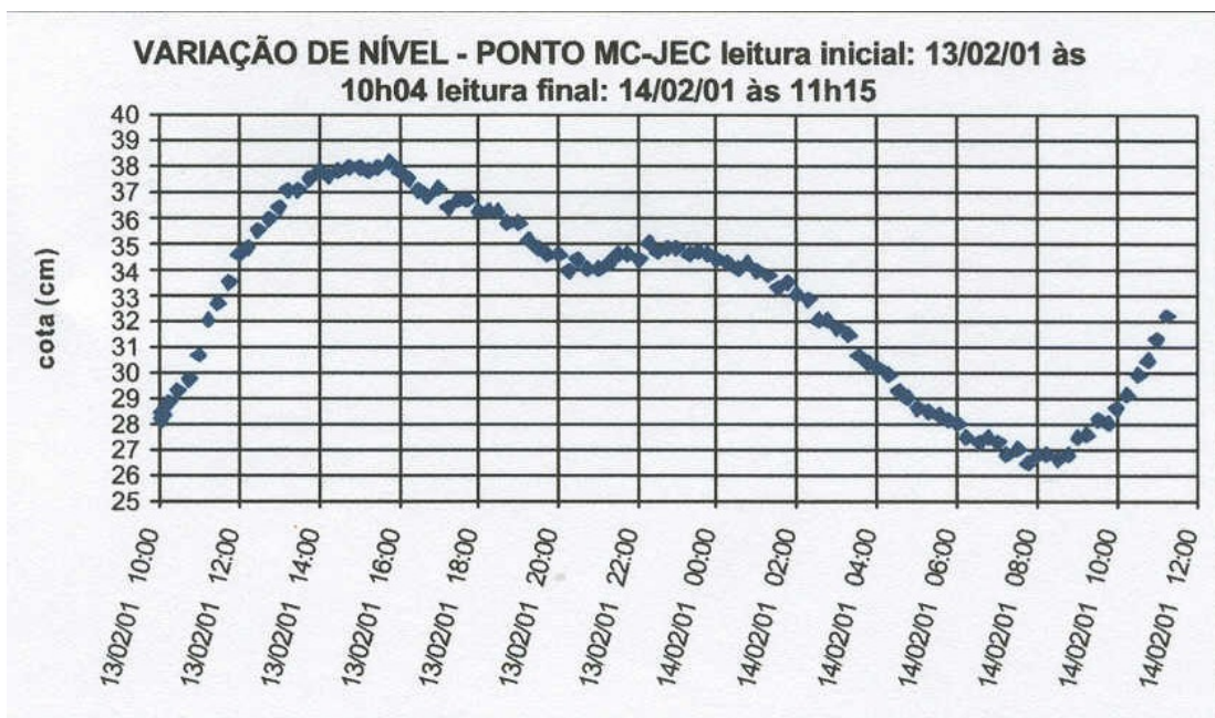
Figura 08 – Medição do nível do rio no ponto MC-JEC ao longo do dia.
