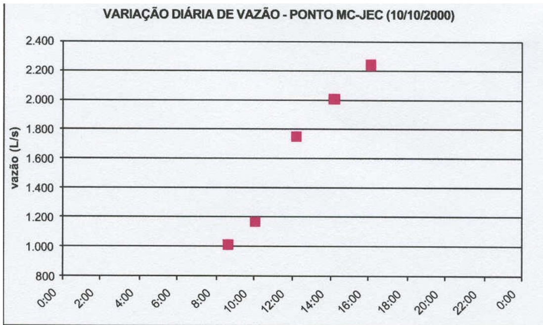
Figura 07 – Variação de vazão no ponto MC-JEC ao longo do dia.
