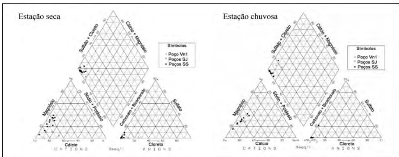
Figura 44 - Diagrama Piper de classificação das águas subterrâneas de São Sebastião (retirado de Santos e Matos, 2006).
