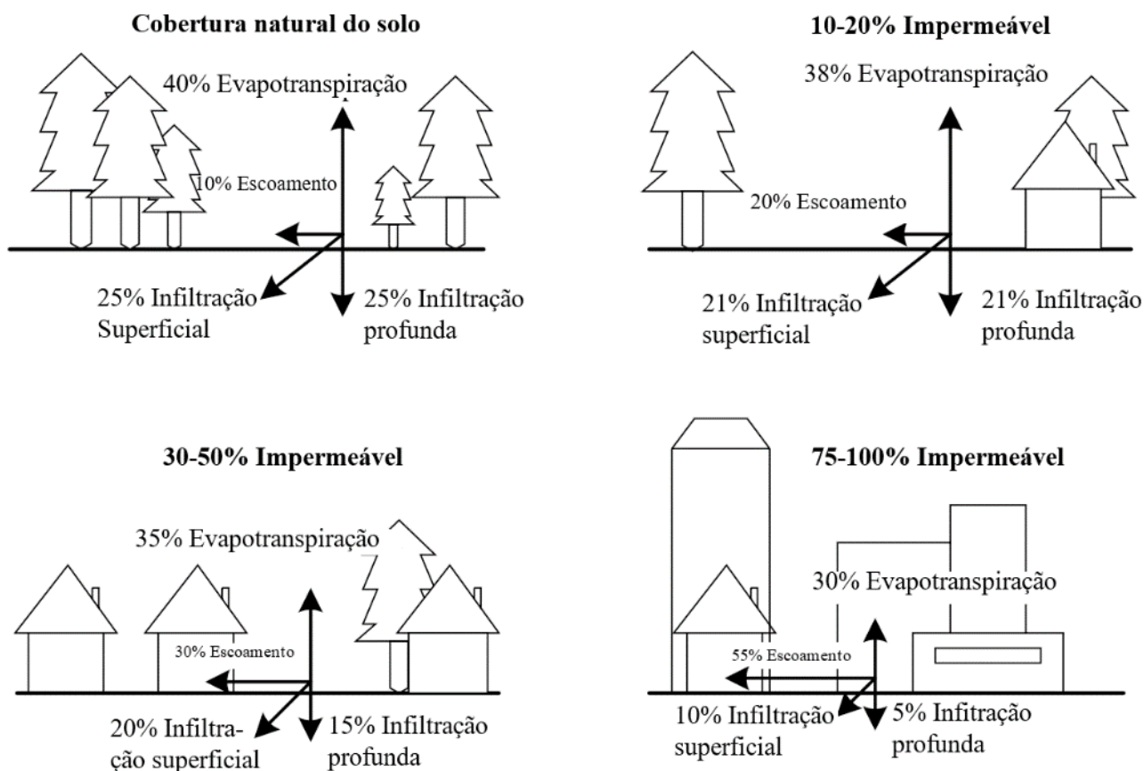
Figura 78 - Efeitos da impermeabilização sobre o escoamento superficial e infiltração. Fonte: Adaptado de Karamouz et al. (2010).
