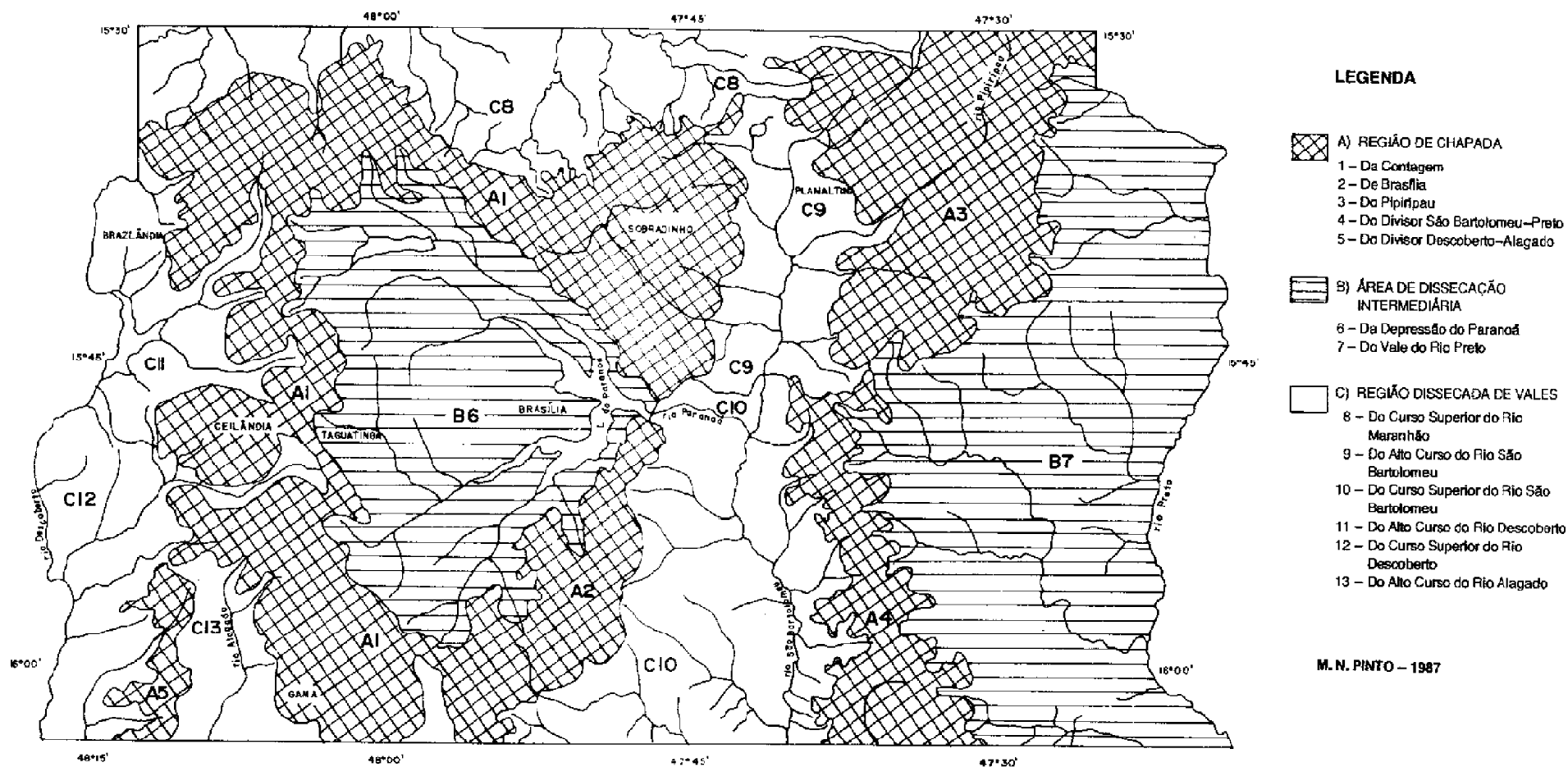
Figura 05 - Mapa Geomorfológico do DF. (Novaes Pinto, 1994)
