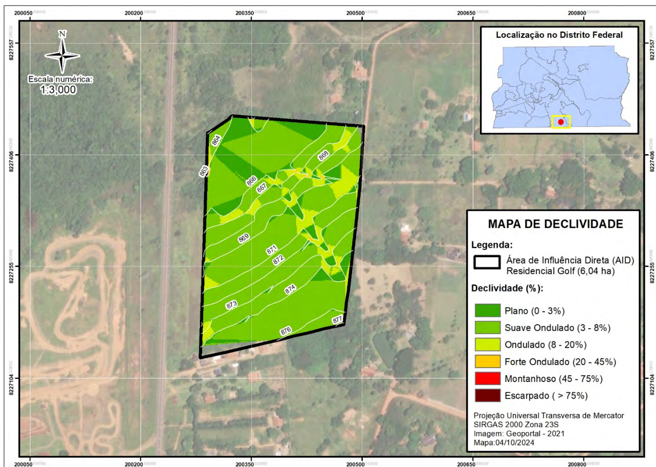
Figura 30 - Mapa de Declividade com base nas curvas de nível obtidas pela topografia. Fonte: TT Engenharia, 2024.
