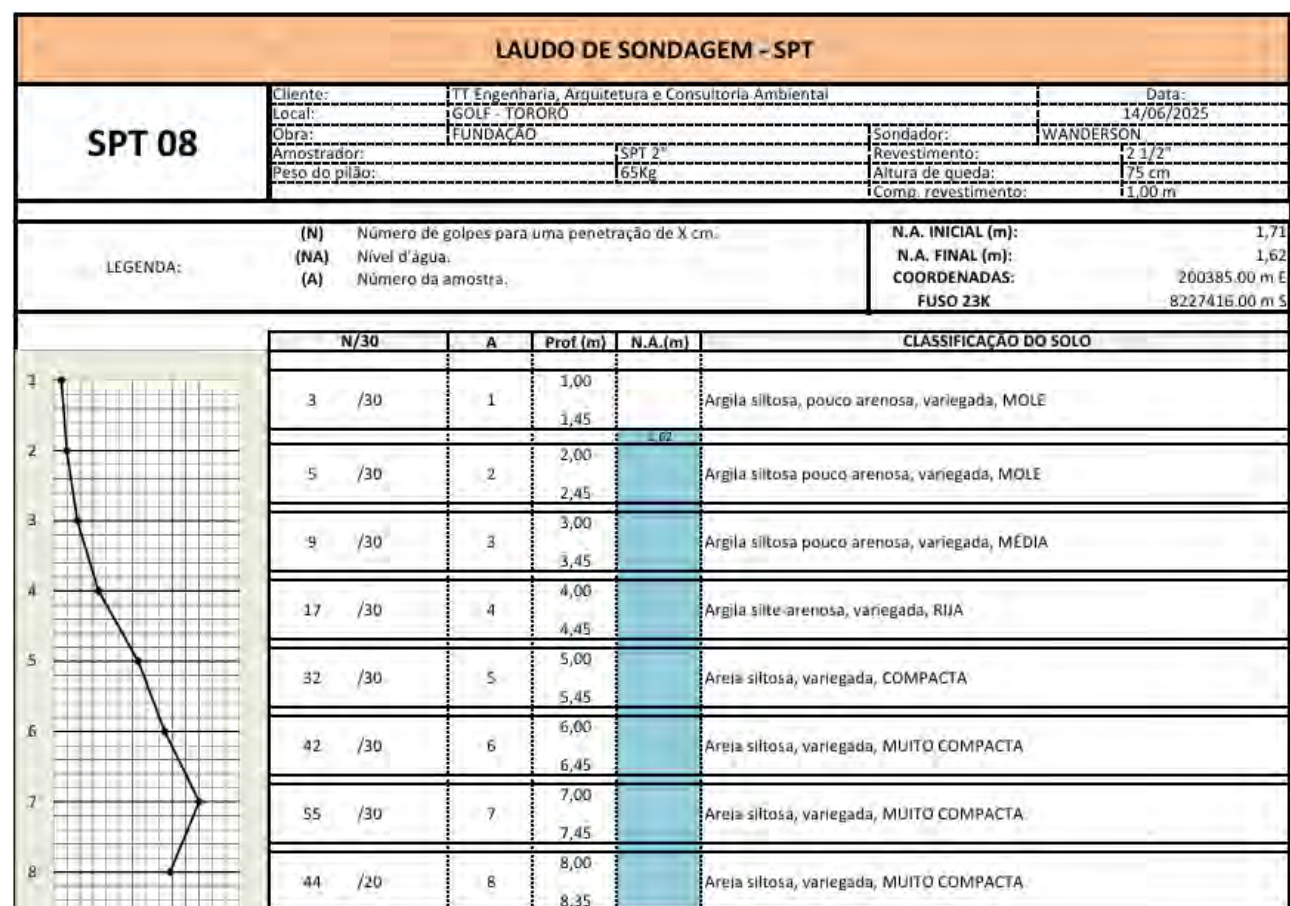
Figura 35 – Laudo de sondagem tipo SPT 08. Fonte: Autor. Documento Original em ANEXO.
