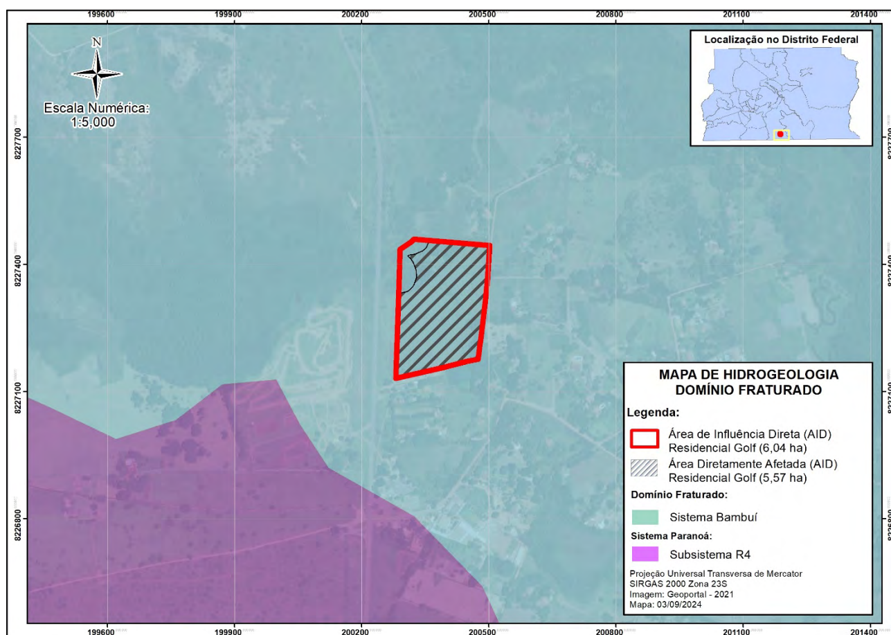
Figura 44 – Mapa da Hidrogeologia do domínio Fraturado. Fonte dos dados: SISDIA, 2023.
