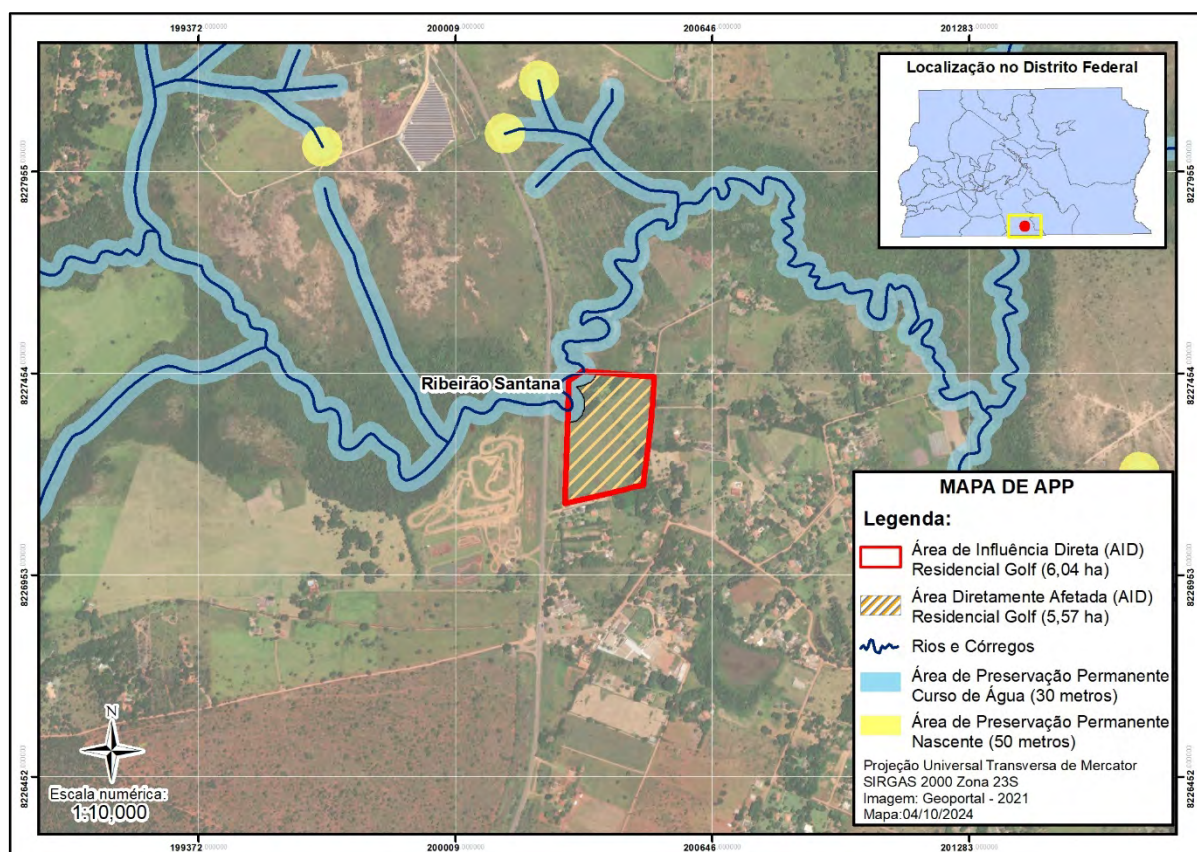
Figura 46 – Mapa dos corpos hídricos, APPs, canais e faixas de proteção. Fonte: vistoria campo e interpretação das curvas de nível topografia.
