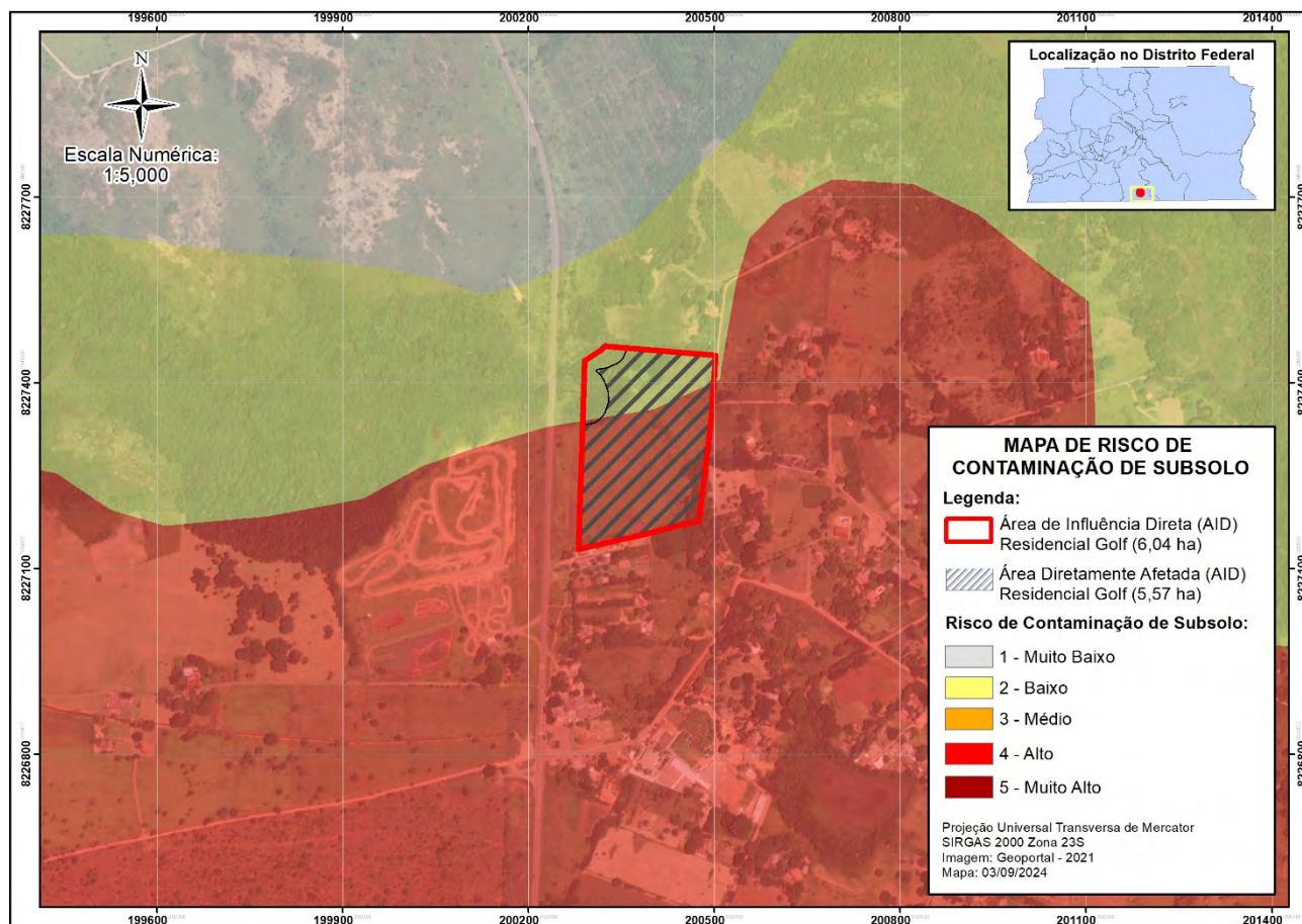
Figura 14 – Mapa de Risco de Contaminação do Subsolo
