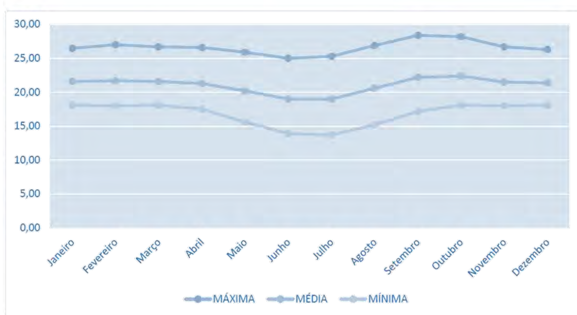
Figura 51 - Temperatura máxima, média e mínima na estação climatológica Brasília. Normais climatológicas (1981-2010) Fonte: INMET.
