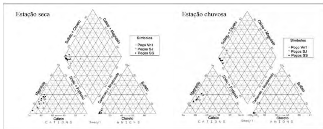
Figura 45 - Diagrama Piper de classificação das águas subterrâneas de São Sebastião (retirado de Santos e Matos, 2006).
