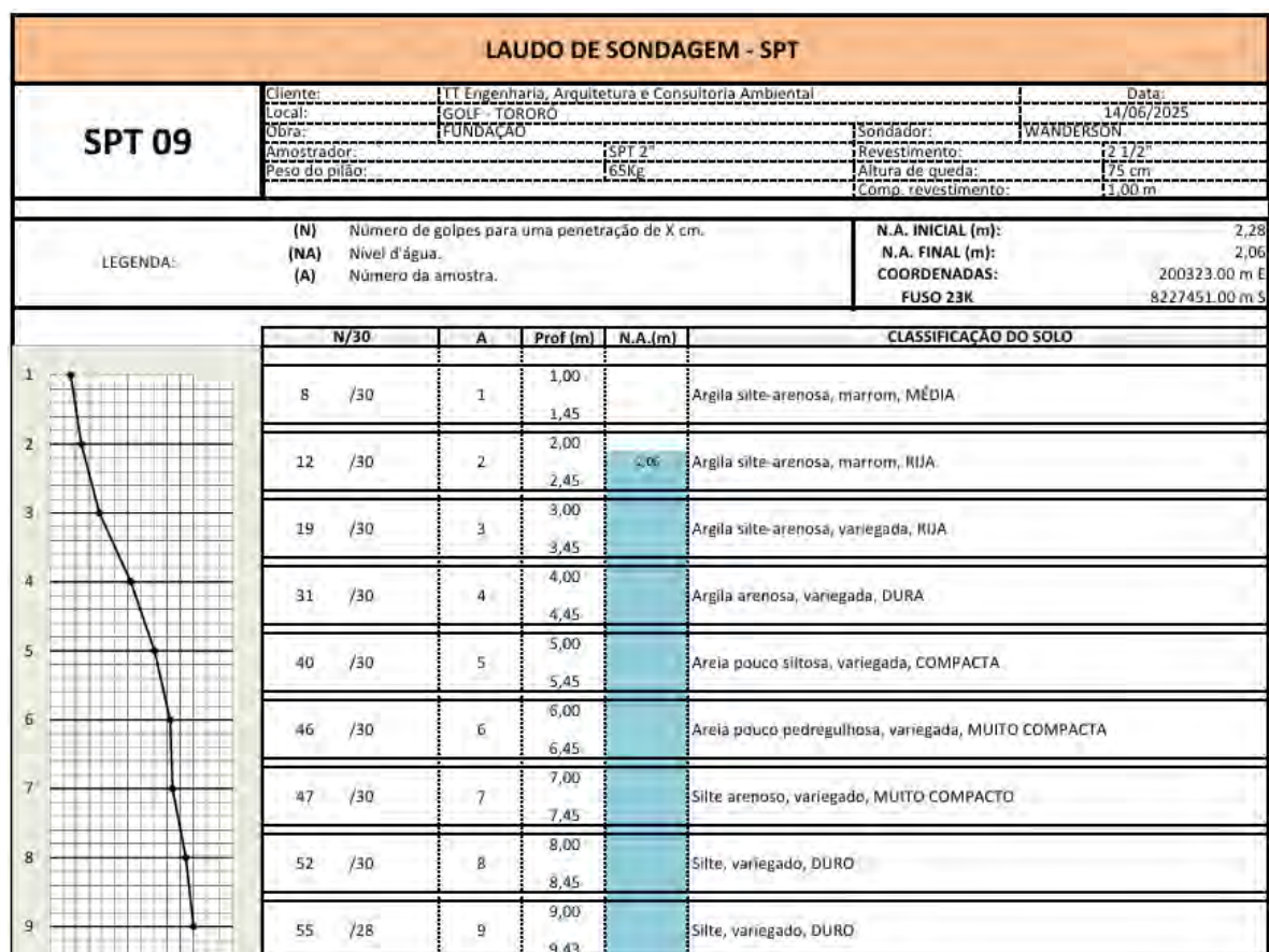
Figura 36 – Laudo de sondagem tipo SPT 09. Fonte: Autor. Documento Original em ANEXO.
