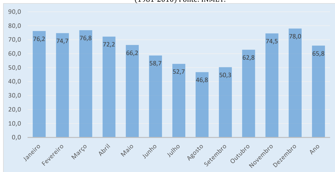
Figura 52 - Umidade relativa na estação climatológica Brasília. Normais climatológicas (1981- 2010 - INMET)
