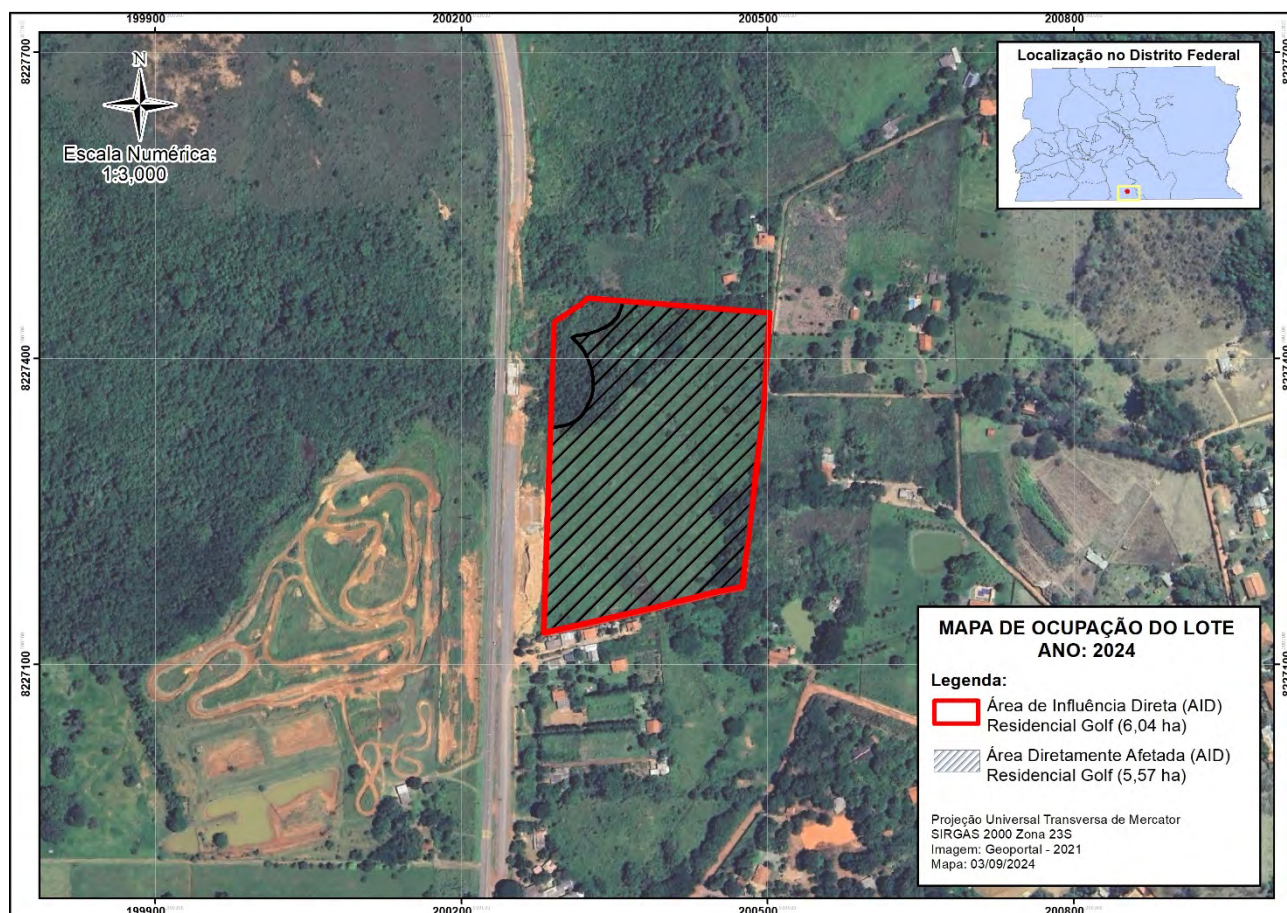
Figura 26- Área do Imovel em 2021. Árvores isoladas e pequena porção de vegetação ao leste.
