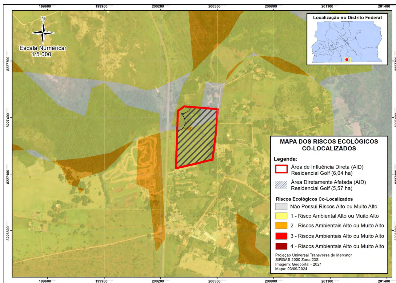
Figura 11 – Mapa de Riscos ecológicos colocalizados
