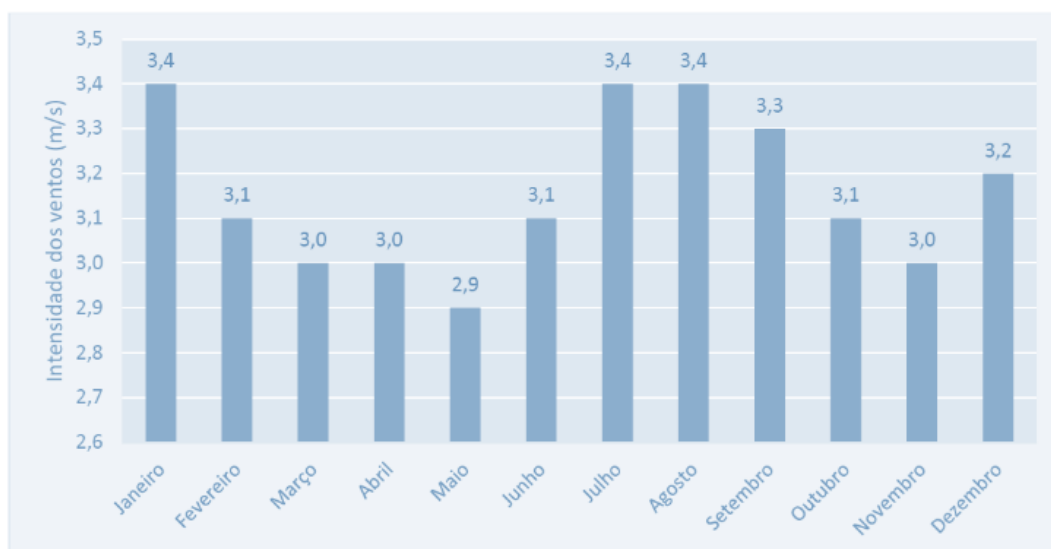
Figura 53 - Intensidade dos ventos na estação climatológica Brasília. Normais climatológicas (1981-2010).
