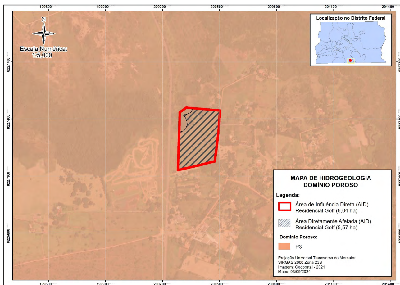
Figura 43 - Mapa Hidrogeológico do DF do domínio poroso na área diretamente afetada. Fonte dos dados: SISDIA, 2023.
