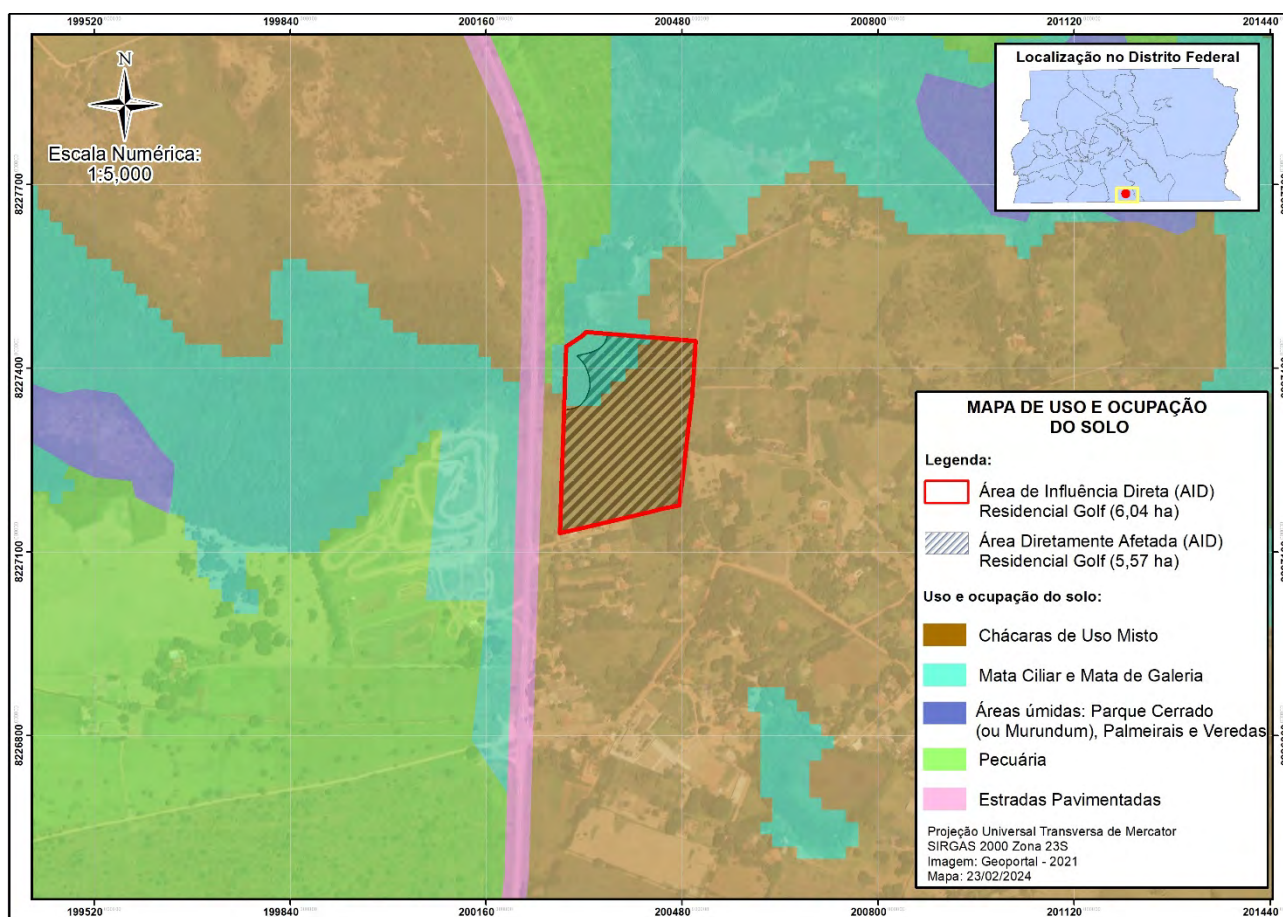
Figura 49 - Mapa de uso e cobertura do solo. Fonte: SISDIA, 2023
