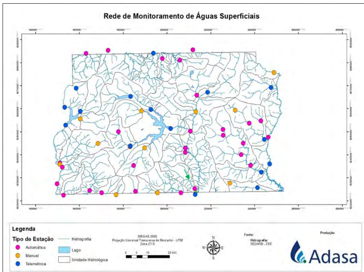
Figura 48 – Mapa da rede de monitoramento da qualidade das águas superficiais. Seta verde indica a Estação de Monitoramento do Ribeirão Santana.
