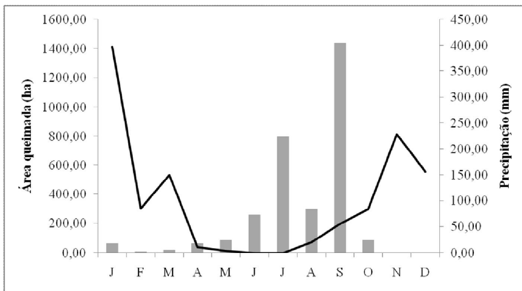
Figura 117. Área queimada (ha) x Precipitação (mm).
