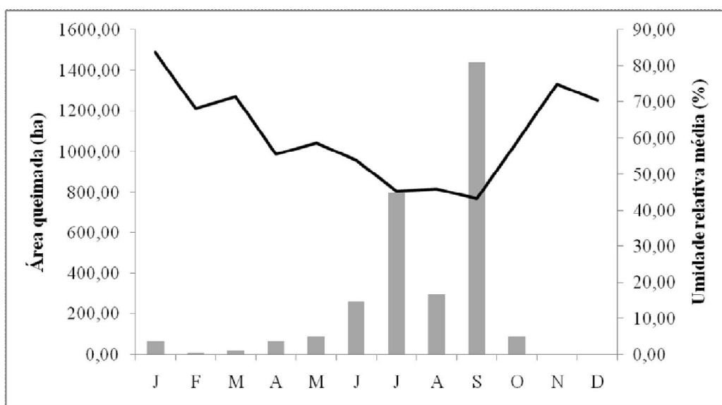
Figura 116. Área queimada (ha) x Umidade Relativa média (%).
